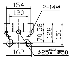
ラム下面
