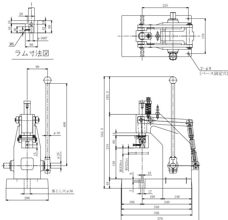
全体図
