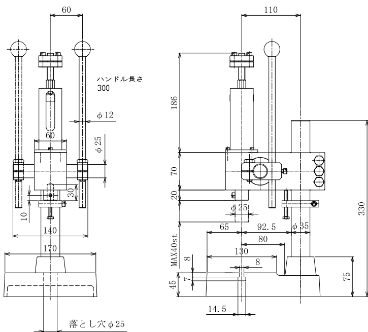
ラム寸法図
