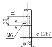
ラム寸法図
