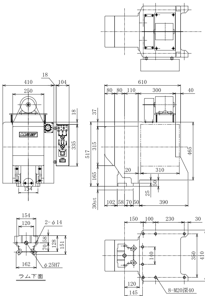
全体図 (BH-55)
