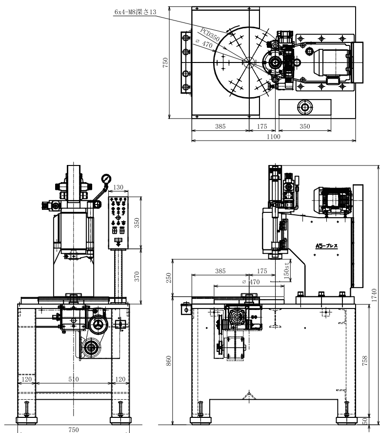
全体図 (AR-5)
